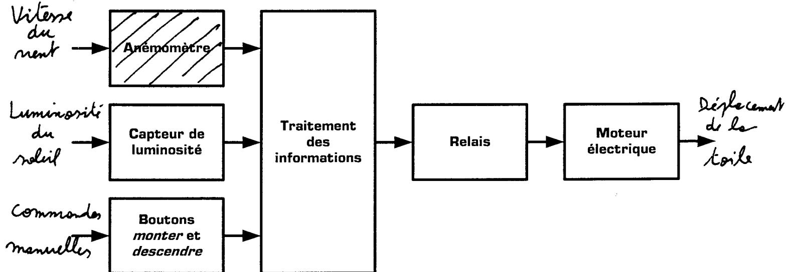
Figure 2 : organisation fonctionnelle du système
