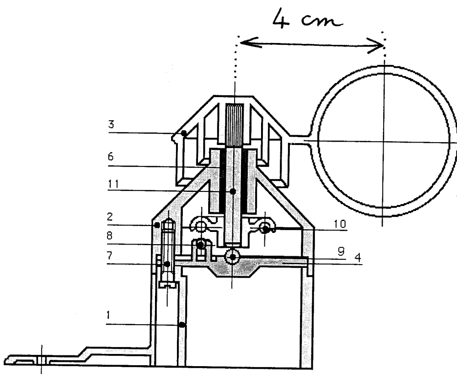
Figure 5 : les 11 éléments principaux de l'anémomètre
