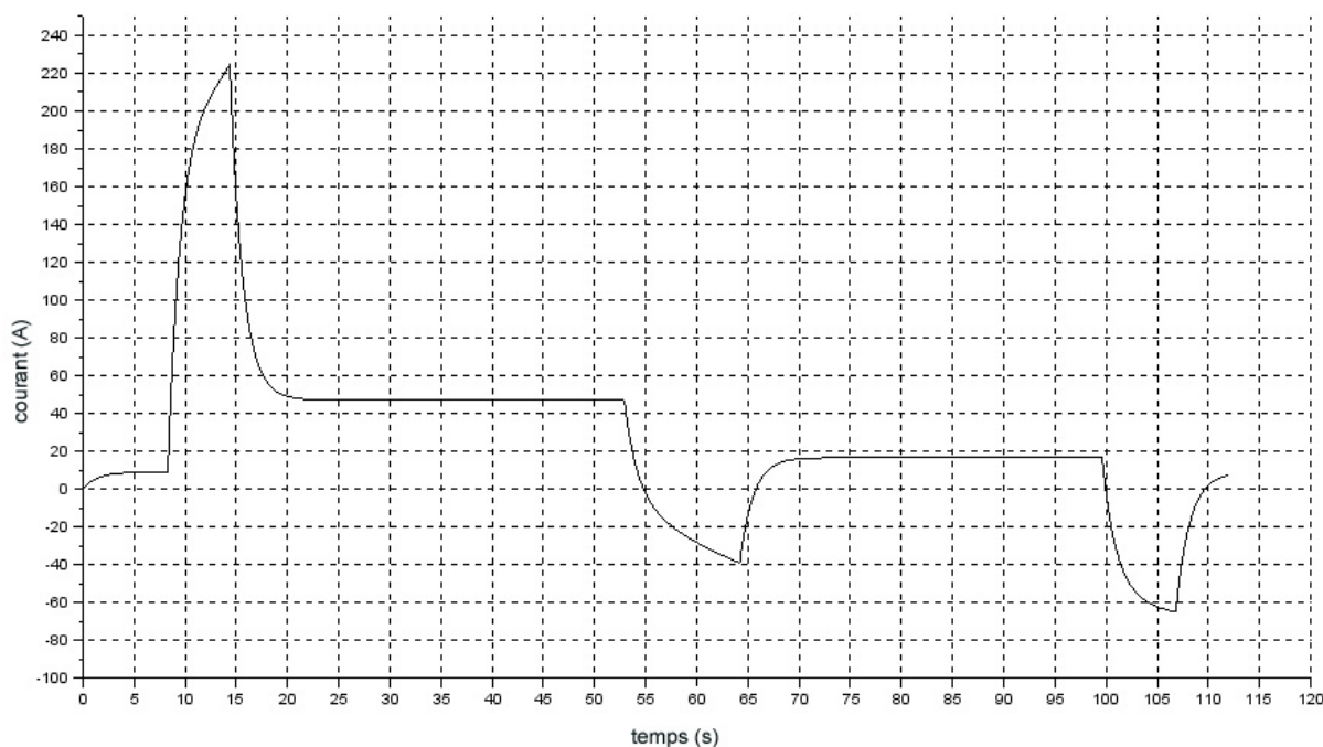
Figure 15 : résultats de la simulation donnant le courant consommé lors d'un cycle ECE 47
