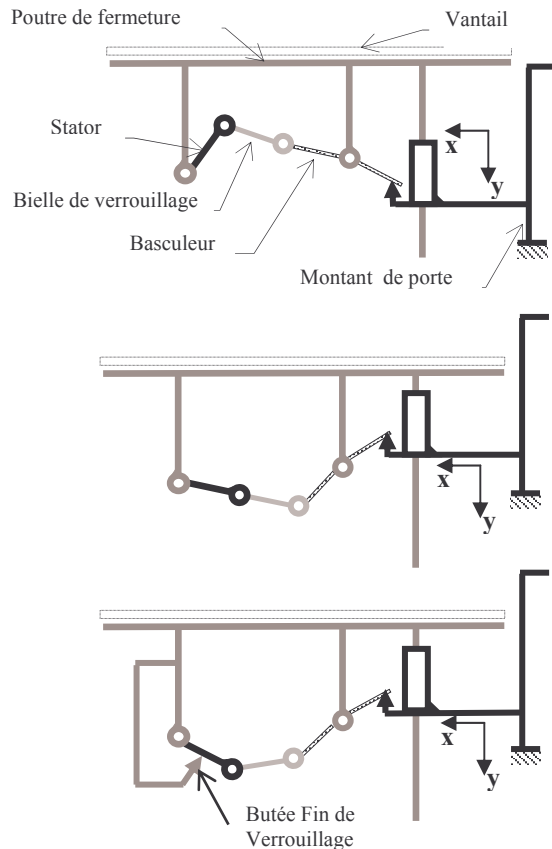
Figure 12 : Schéma cinématique
