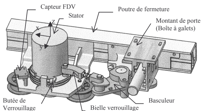
Figure 10 : Verrouillage dessus
