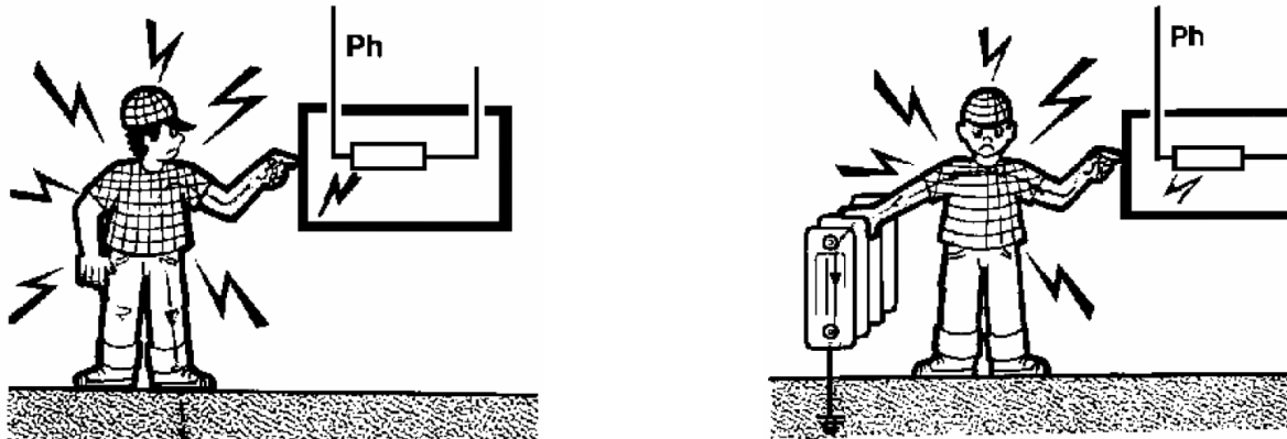
Contact indirect : l'utilisateur touche la carcasse métallique d'un appareil, mais cette carcasse était sous tension
